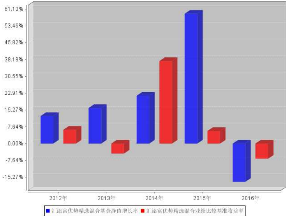
汇添富优势精选混合过去五年基金每年净值增长率及其与同期业绩比较基准收益率的对比图
