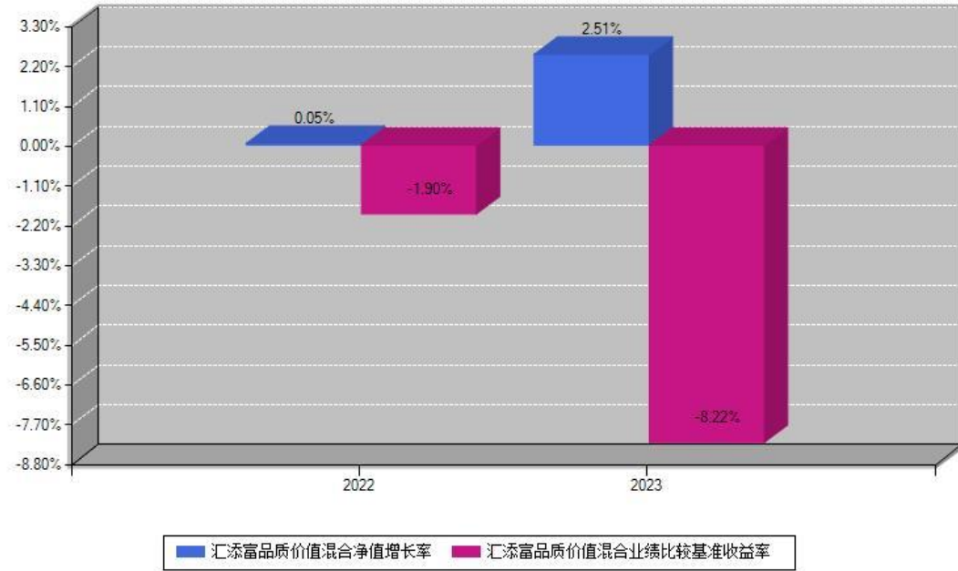
汇添富品质价值混合每年净值增长率与同期业绩基准收益率对比图
